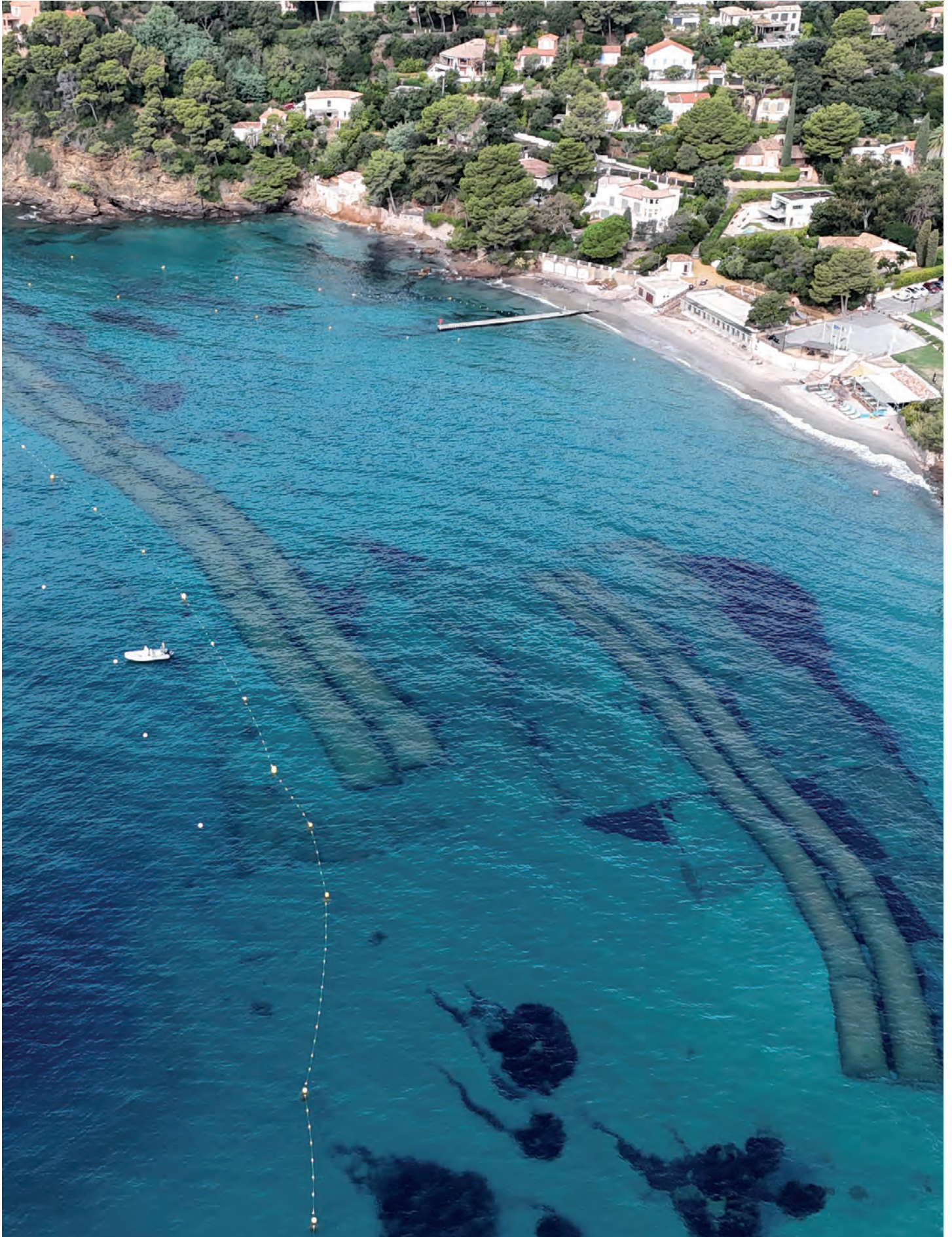
Les géotubes – Plage du Rayol
